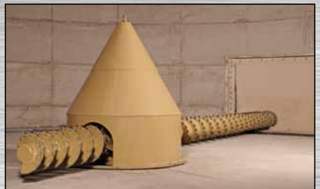
环形驱动筒仓回收装置
